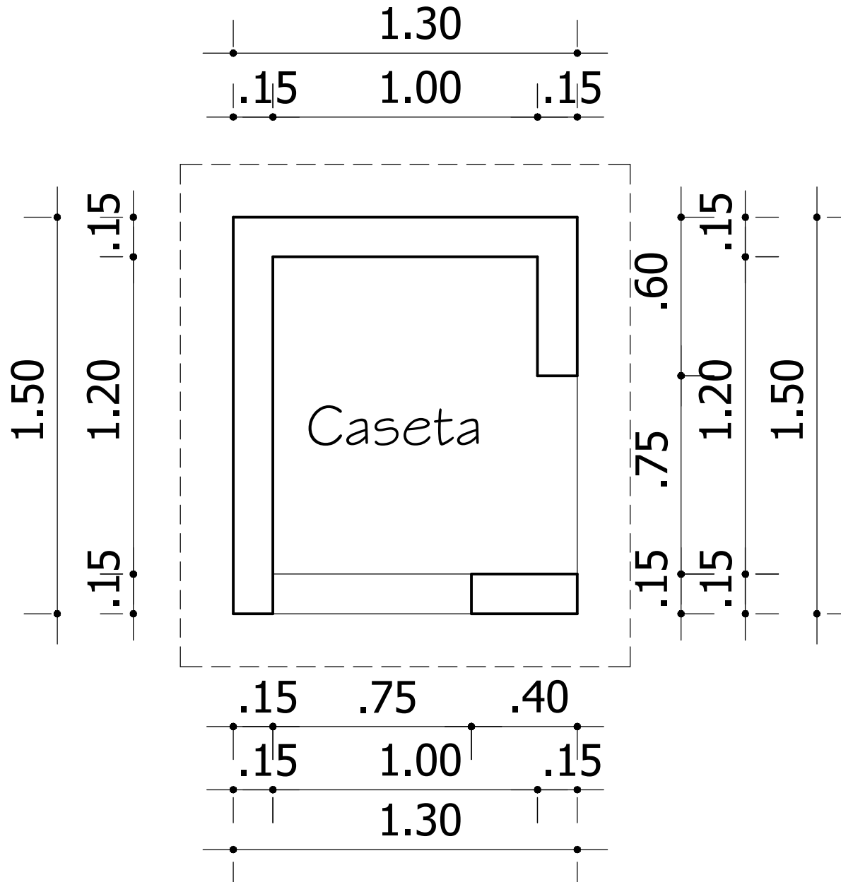
Planta Dimensionada
